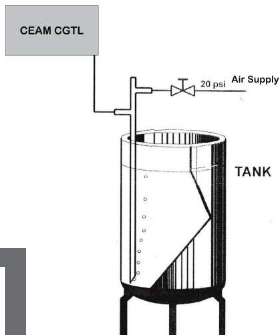
Nella Foto Dx: Esempio applicativo del CGLT-01
